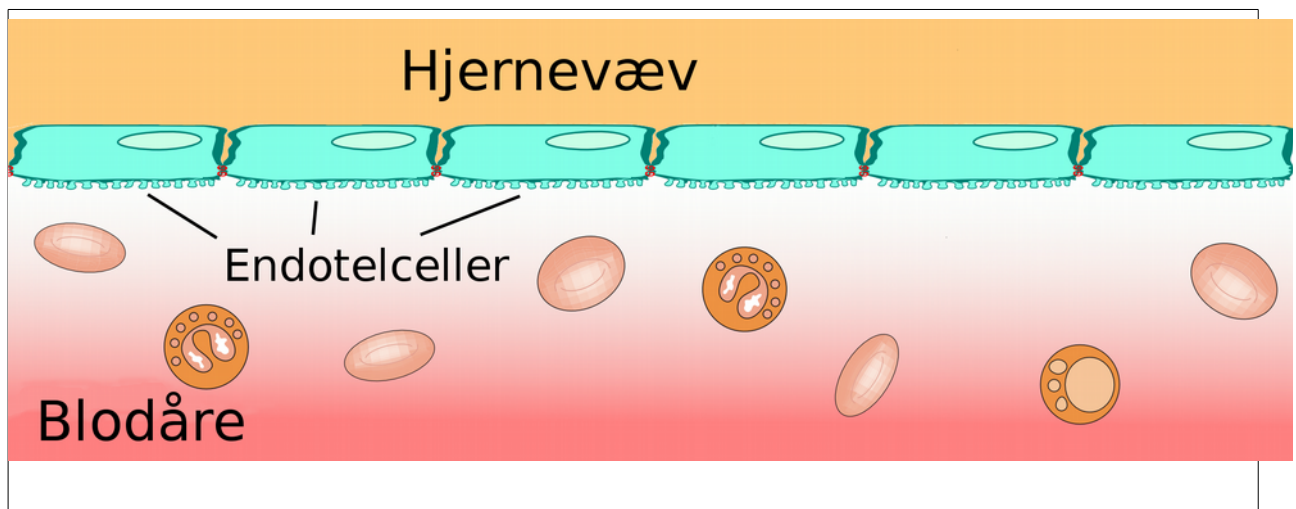
Figur 28: Principskitse for blod-hjerne-barrieren. Bemærk sammenkoblingen mellem endotelcellerne som udgør blod-hjerne-membranen. Illustration: Bearbejdning af materiale fra Wikimedia Commons.
